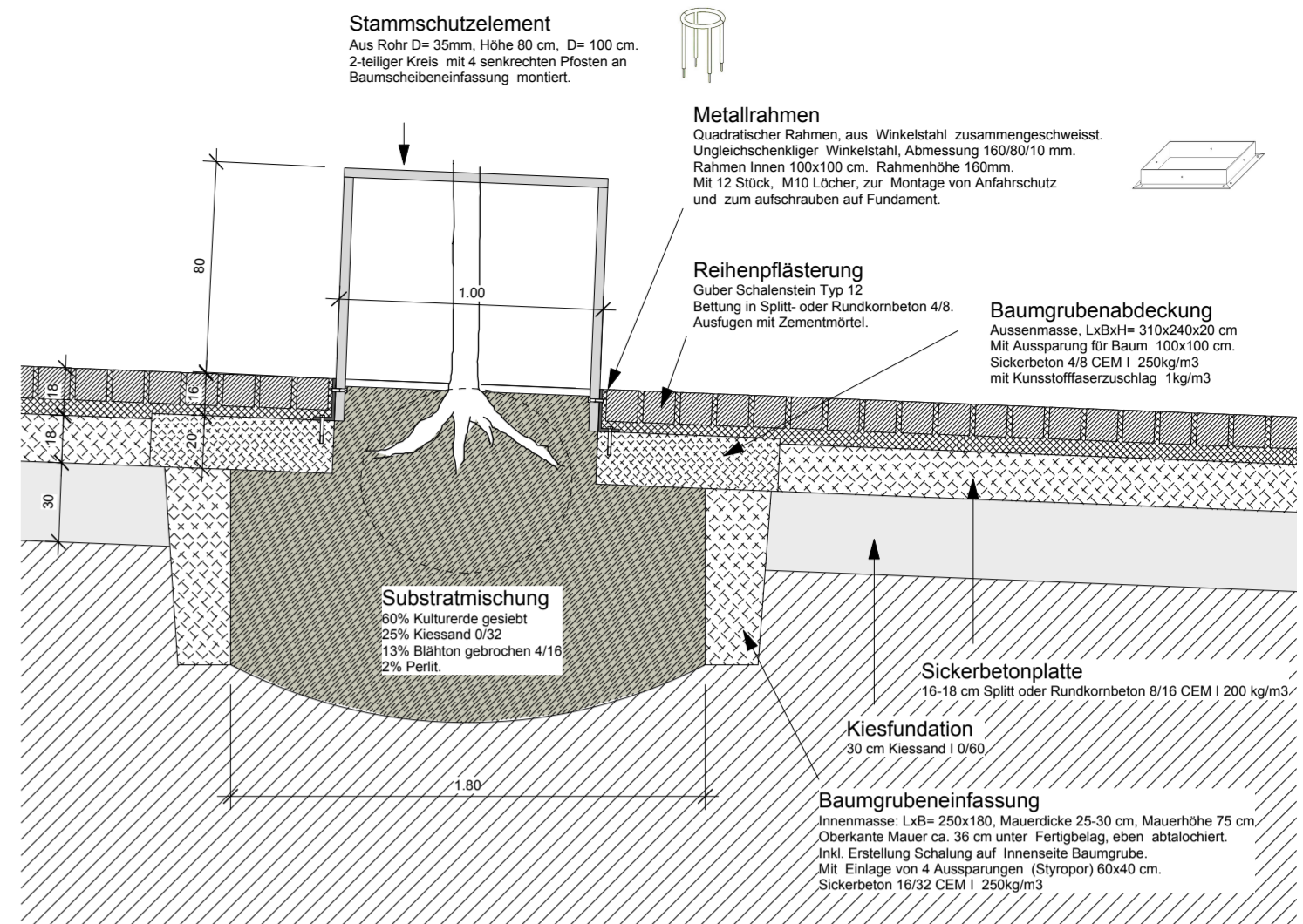
Schemaschnitt Baumgrube 1:25
